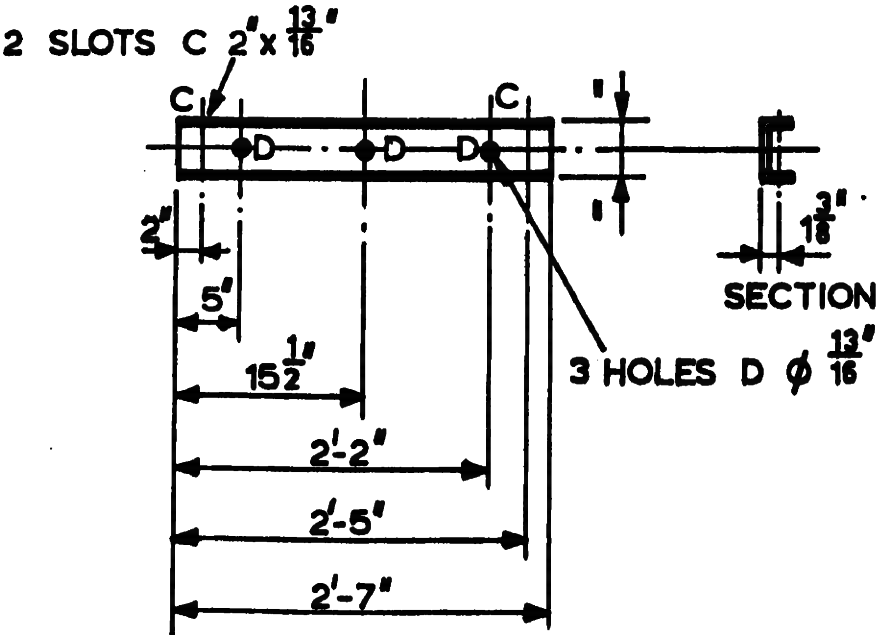
ELEVATION ITEM ②
