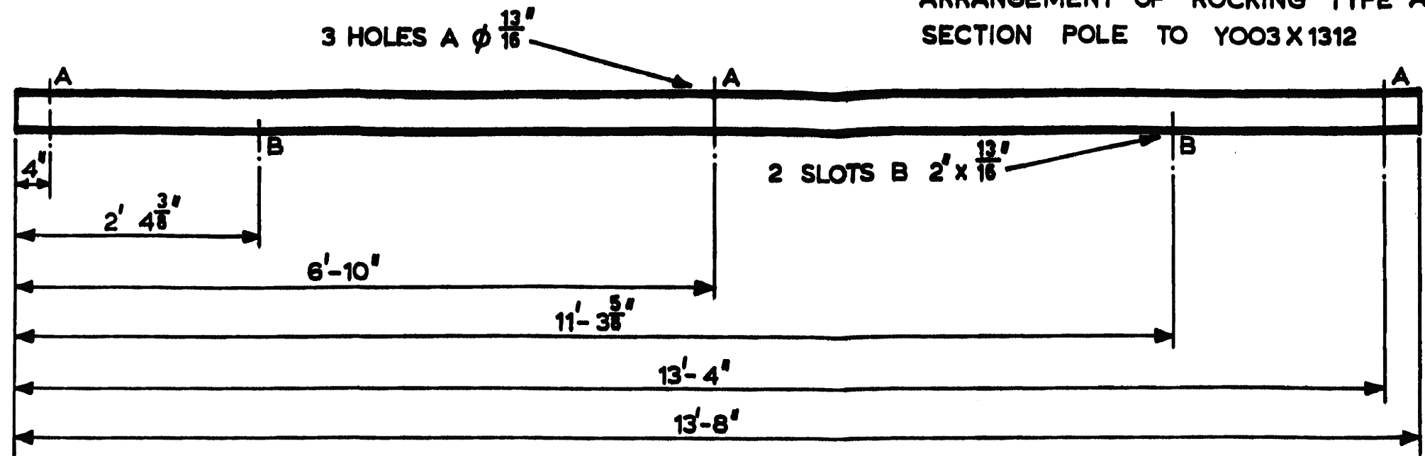
ELEVATION ITEM ①
